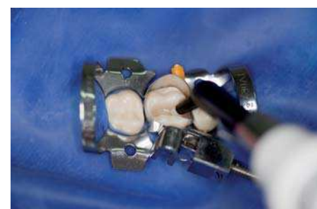
Appliquer une couche de 2 mm de GrandioSO
