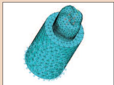
Рис. 5. Объединенная модель коронки, имплантата и кости (программа для FEA).
