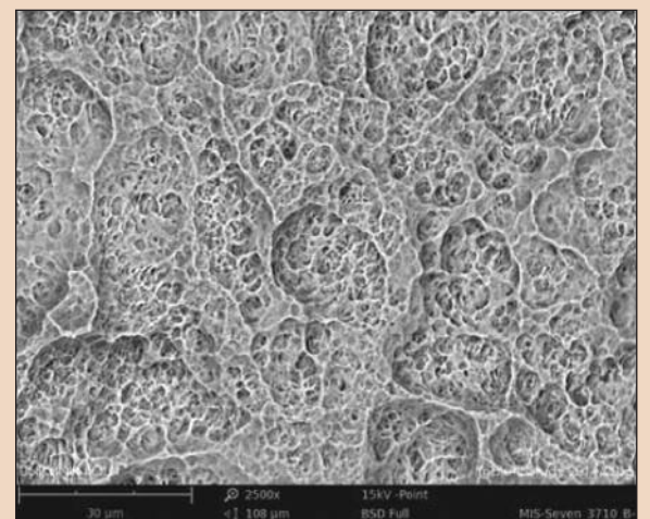
Слева: чистая поверхность имплантата MIS Seven (ув. 500). Справа: микро- и наноструктура поверхности имплантата (ув. 2500); фотографии: доктор Dirk Duedeck и доктор Jörg Neugebauer, Кельнский университет.
