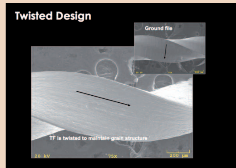
Рис. 2. Структура файла TF в сравнении с инструментом, изготовленным методом вытягивания.
