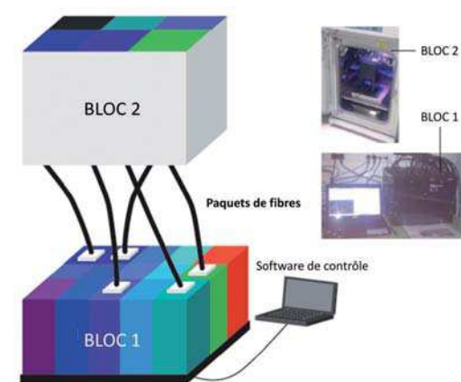
Fig. 5 : Le modèle photométrique est un système d'illumination fibré à LED qui permet de mesurer de manière rigoureuse le calcul de l'éclairage rétinien et développer un système spécifique d'illumination cellulaire.
