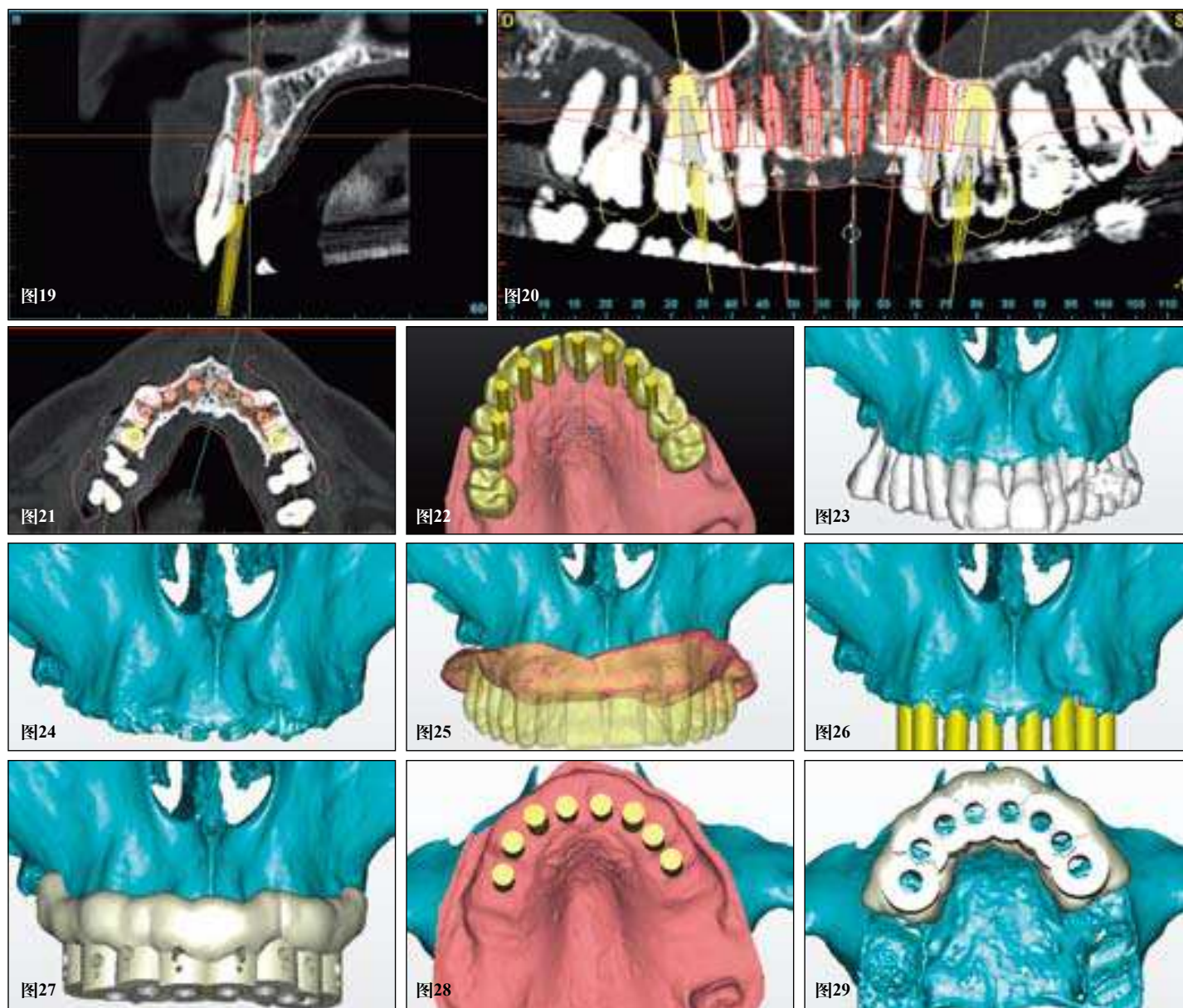
图19: 牙齿和植入种植体的横断面观。 图20: 曲断展示整个治疗方案。 图21: 治疗计划的纵断面观。 图22: 虚拟三维观: 对于该较重的病例比较难理解,而且最终的结果并不一定更好,因此并没有使用虚拟设计。 图23: 在设计软件中观察到的将要拔除的牙齿,以及骨结构。 图24: 在设计软件中观察牙齿拔除后的状况。 图25: 在设计软件中扫描、匹配改进状况。这里可以看到牙龈和骨结构。通过该设计中的模型数据可以达到此目的。 图26: 种植体轴的平行延长。 图27: 软件中有骨支持的SIMPLANT SAFE导板。 图28: 三维模型的虚拟模板。 图29: SIMPLANT SAFE导板的虚拟模型。
