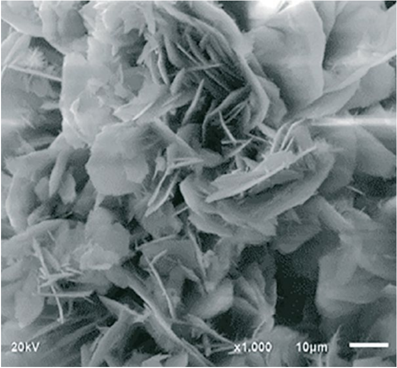
Afb. 1 Na contact van calciumsilicaatcement met calcium- en fosfaationen uit lichaamsvloeistoffen vormt zich een hydroxyapatietachtige neerslag op het oppervlak. Hier in vitro gesimuleerd door Biodentine (Septodont) gedurende zes maanden te bewaren in een fosfaatgebufferde zoutoplossing (PBS). Het beeld op de elektronenmicroscopische opname is 1000× vergroot.
