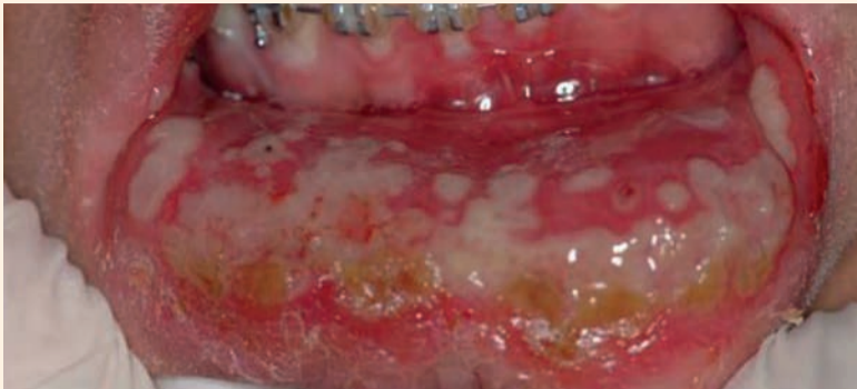
Fig. 15 - Herpes labialis.
