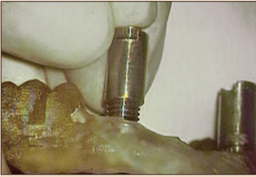
Рис. 7з. Устройство в сборе на хирургическом шаблоне (клинический случай 1).
