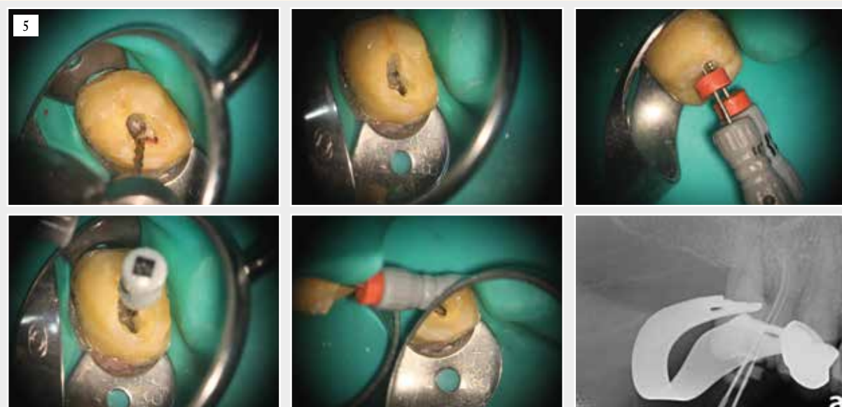
Fig. 5: L'évaseur One Flare® assure une élimination des premiers mm du parenchyme pulpaire et libère les contraintes sur les limes qui sont recentrées dans le canal pour faciliter l'accès et la mise en forme à la limite apicale de préparation.
