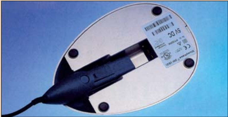
Εικ. 14Ο χρόνος αναμονής λόγω εξαντλημένης μπαταρίας εξαλείφεται λόγω της λειτουργίας Click&Cure. Για μία ομαλή εργασία στο οδοντιατρείο, η χειρολαβή μπορεί να συνδεθεί με καλώδιο ρεύματος της βάσης φόρτισης οποιαδήποτε χρονική στιγμή.
