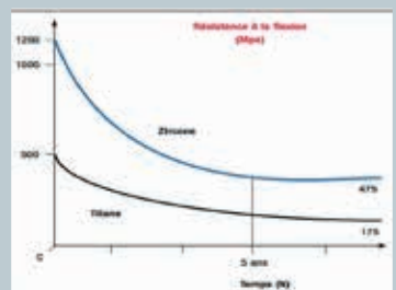
Fig. 5: Résistance à la flexion de la zircone comparée au titane.
