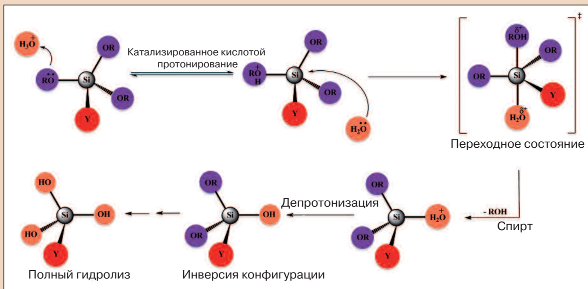
Рис. 1. Механизм гидролиза силиана.
