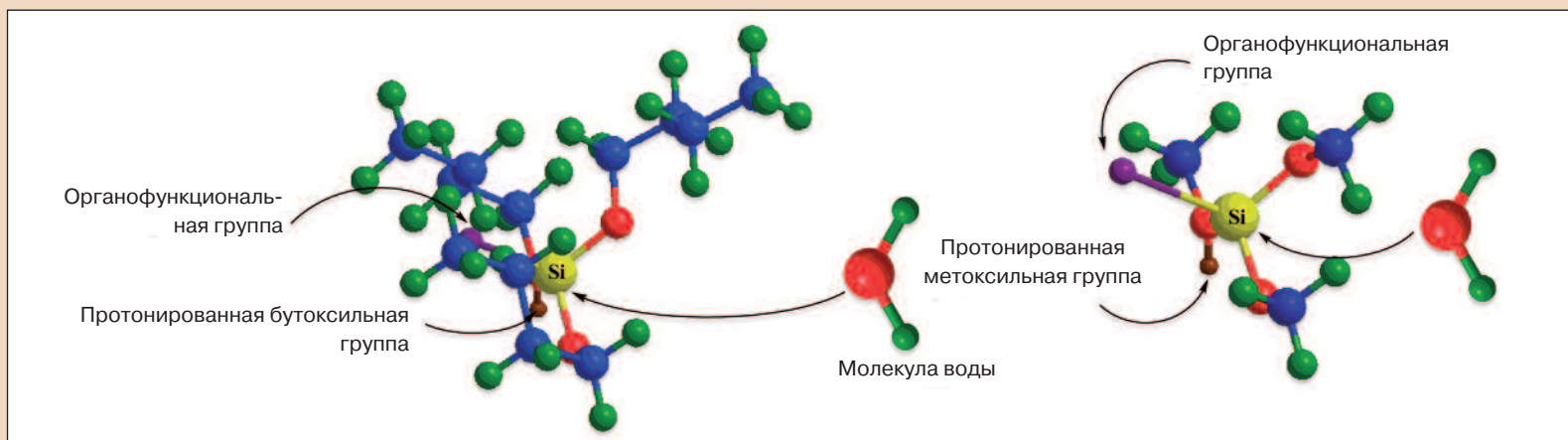
Рис. 2. Стерическое воздействие алоксильных групп на гидролиз силиана; шаростержневая модель различия между метоксильной и бутоксильной группами.
