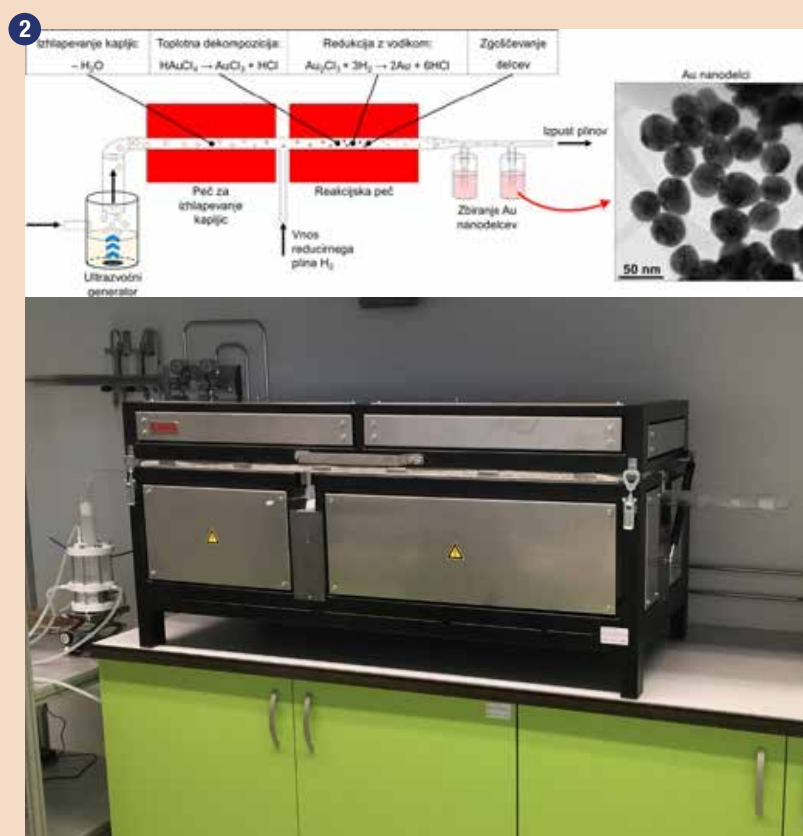
Shema nastanka zlatih nanodelcev pri USP, predstavitev nanodelcev in postavitev naprave USP v Zlatarni Celje d.o.o. (foto: ŽC)
