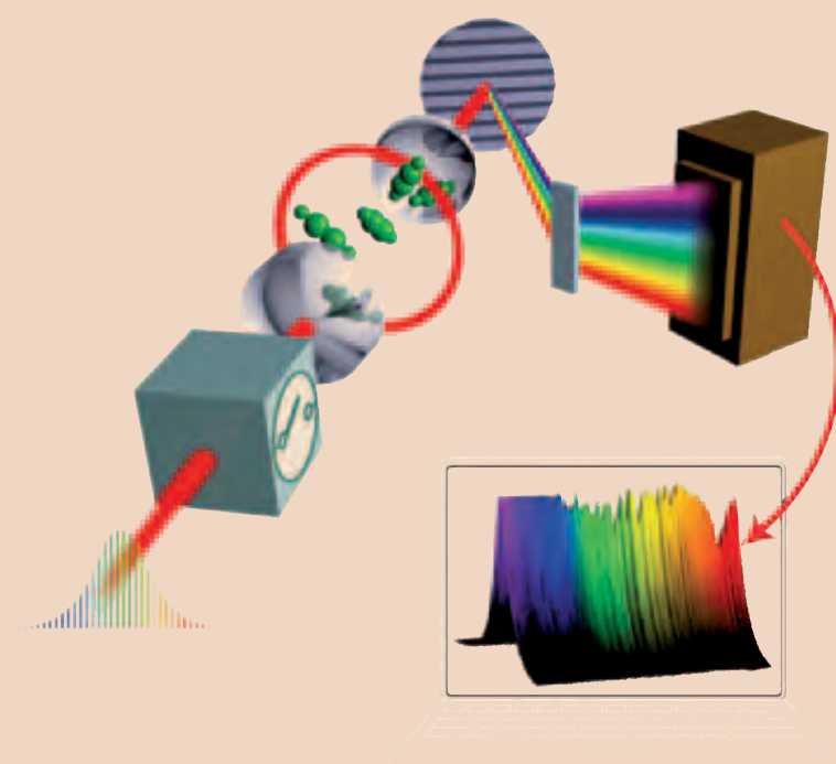
Ryc. 2. Wzmocniona laserowa spektroskopia optyczna z zastosowaniem różnych częstotliwości umożliwia jednoczesne wykrywanie wielu cech w szerokim spektrum z wysoką czułością i rozdzielczością; Ryc. Jeff Fal, JILA.
