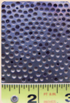
Der Kompositmetallschaum im Maßstab (Foto: NCSU, USA).
