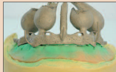
Рис. 18. С помощью маркерного спрея проверили супраструктуру на наличие областей трения и неправильных контактов, чтобы обеспечить пассивность ее посадки на балке.
