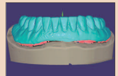
Рис. 6. С помощью акрилового шаблона определили правильное расположение восковой модели относительно имплантатов, затем провели сканирование набора зубов и модели с размеченными имплантатами.
