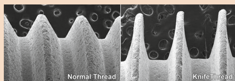
Mikroskopski pogledi na standardno V-oblikovano zasnovo navojev (EZ Plus Internal; levo) in novejšo zasnovo z nožastimi navoji (AnyRidge; desno).
