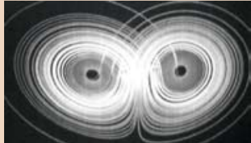
Фиг. 5. Атрактор на Лоренц. Изследване, базиращо се на математически анализ на слож-
