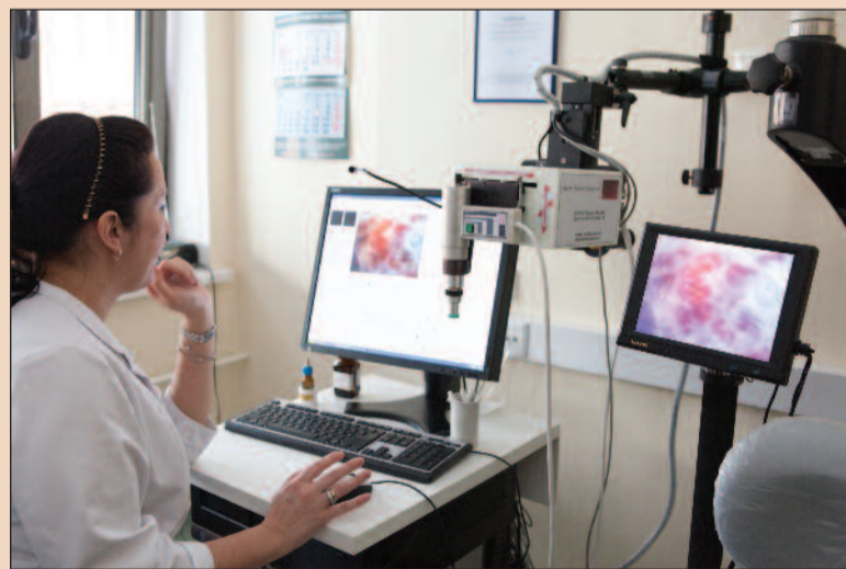
Аппаратура для проведения компьютерной капилляроскопии.
