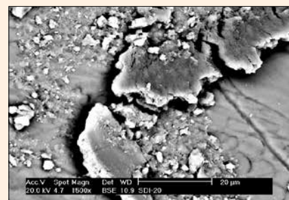
Imagen de microscopio de barrido a 1500 y 3000 aumentos, donde se observa la ruptura de los cristales del esmalte después del uso de Pola Office (SDI) durante 20 minutos en 3 aplicaciones, más lámpara Zoom.
