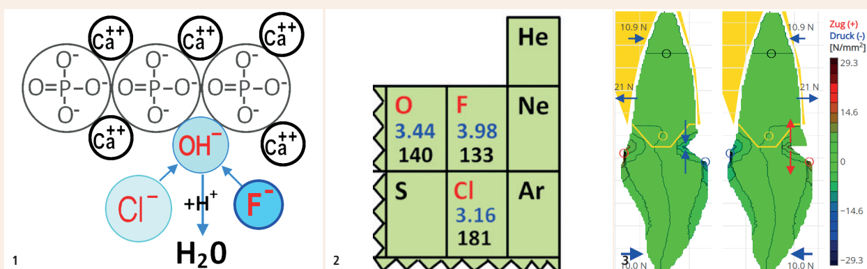
Abb. 1: Der Ionenaustausch beim Hydroxylapatit. – Abb. 2: Ausschnitt aus dem Periodensystem (mit Elektronegativität und Ionenradius). – Abb. 3: links: Eine normale Kaukraft setzt den Zahnhals unter Druck (blauer Doppelpfeil); rechts: Der Zug (roter Doppelpfeil) stoppt bei einem Mikroriss im Kerbgrund.
