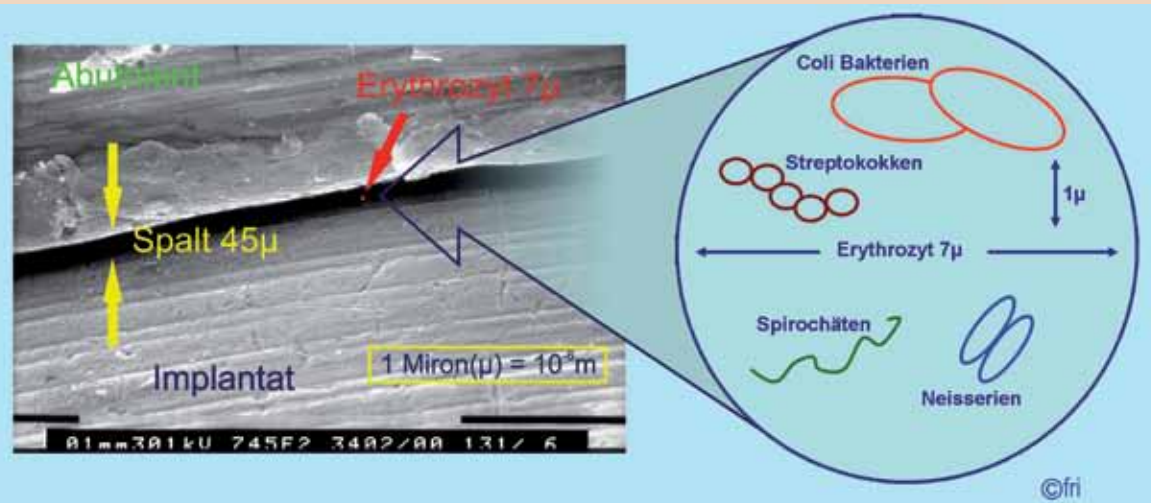
Ryc. 4: Szczelina między implantem i łącznikiem w stosunku do erytrocytów o średnicy 7\mu ( \mu = 10^{-6} m), powiększenie 745 x, losowo wybrane bakterie podane do skali w porównaniu do erytrocytów.
