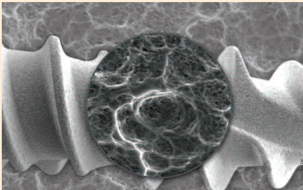
Fig. 2 : Surface de l'implant Alpha-Bio Tec (Microscope électronique à balayage x 20 et x 1 000)
