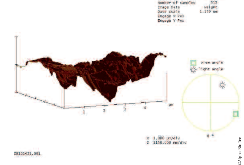
Fig. 1 : Rugosité de la surface de l'implant Alpha-Bio Tec
