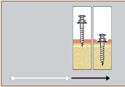
사진. 2.7a & b: Thread mechanisms를 보여주는 도표: self-cutting형과 self-tapping형.
