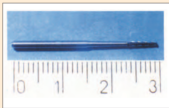
► Fig. 1 : « Fresissima » le corps et la partie active sont tous deux constitués d'un monobloc de carbure de tungstène.
