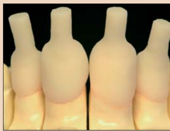
Рис. 5. После удаления реакционного слоя коронки из материала IPS e.max Press демонстрируют превосходную подгонку.
