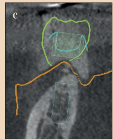
Resim 11a: Durum modeli STL ağı (kırmızı) ve wax-up (yeşil) planlanmış implant ve abutment ile. Resim 11b: Cerrahi kılavuz üretimi için olan çoğaltma modelinin tasarlanmış delme kovanları ile STL ağı. Resim 11c: Planlanmış implant ve kovan konumu ile ortogonal kesit regio 45; turuncu çizgi: durum modeli yüzey profili (dişeti); yeşil hat: Yüzey kontürü wax-up; aqua hattı: delme şablonunun gerçek yüzeyi.
