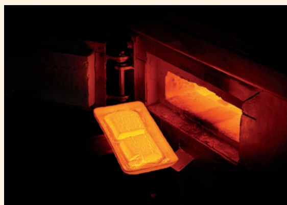
2. ábra: A felhevített massa eltávolítása az égetőkemencéből 1000 °C-on. Ezt követően baziskerámia gyártására használják.
