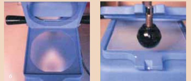
Εικ. 6 Τα φύλλα τοποθετούνται στο συγκρατητήρα. Στη συνέχεια ο συγκρατητήρας κλείνει και σφίγγουμε τη βίδα για σταθερή συγκράτηση του φύλλου.
