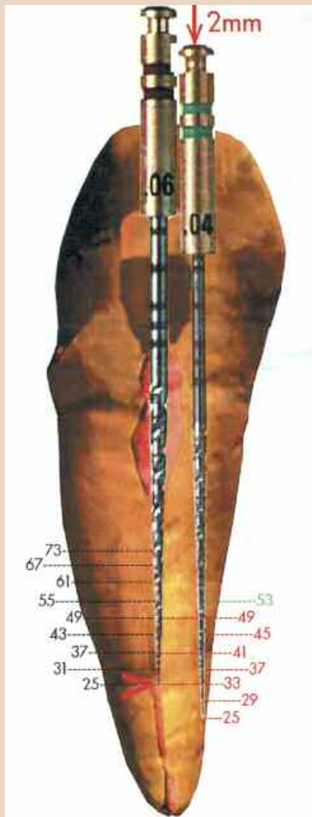
Εικ. 1. Αν η ρίνη 25/0.04 προωθηθεί μόνο 2χιλ. πέρα από το πέρασμα της παροσκήνης της ρίνης 26/0.06, γίνεται ενσφήνωση σε 7 χιλ του σωλήνα.
