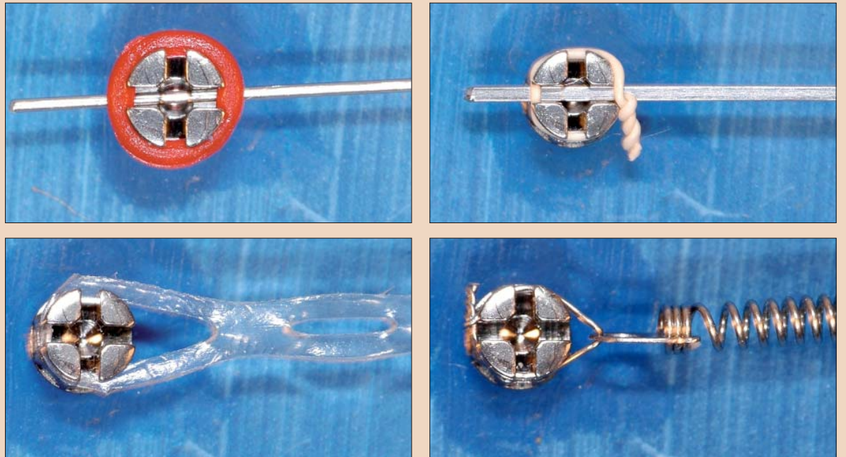
사진. 1.8: 실제적인 이유로 인해, 오직 한개의 보편적으로 적용가능한 헤드 variant를 제공하는 시스템을 사용하도록 권장된다. 이러한 싱글 헤드들은 모든 종류의 결합 장치의 사용이 가능하다 (threads, elastic chains, round wires, square wires).
