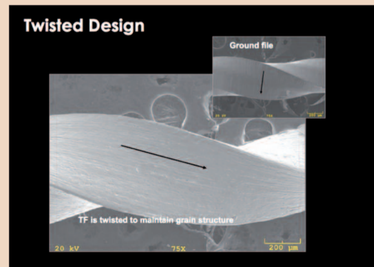
Рис. 2. Структура файла TF в сравнении с инструментом, изготовленным методом вытравливания.
