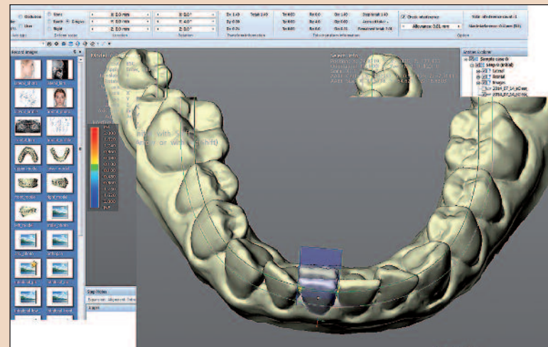
Рис. 6. Программа для трехмерного моделирования eClinger обеспечивает полный контроль перемещения каждого зуба. Сегмент выделяется и преобразуется в куб с регулируемым центром вращения.
