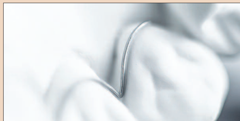
Рис. 14. Увеличенное изображение ретейнера Memotain после электролитической полировки. Края проволоки, сохраняющей квадратное сечение, закруглены.
