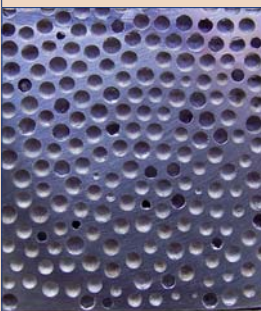
Увеличенное изображение композитной металлической пены (ДП) (фото любезно предоставлено NCSU, США).
