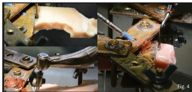
Fig. 4 - Valutazioni fisiche ex vivo su osso di calvaria suina. Mediante una termocoppia vengono rilevate le variazioni di temperatura durante l'esecuzione di osteotomie per la preparazione dei tunnel implantari. In alto a sinistra la sistemica piezoelettrica, in basso le frese con stop di profondità, a destra gli inserti sonici per la preparazione del sito implantare.
