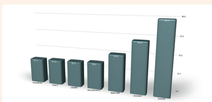
Figure 10 : mesure de déviations du test in-vitro arcade complète avec préparations dentaires et scanmarkers
