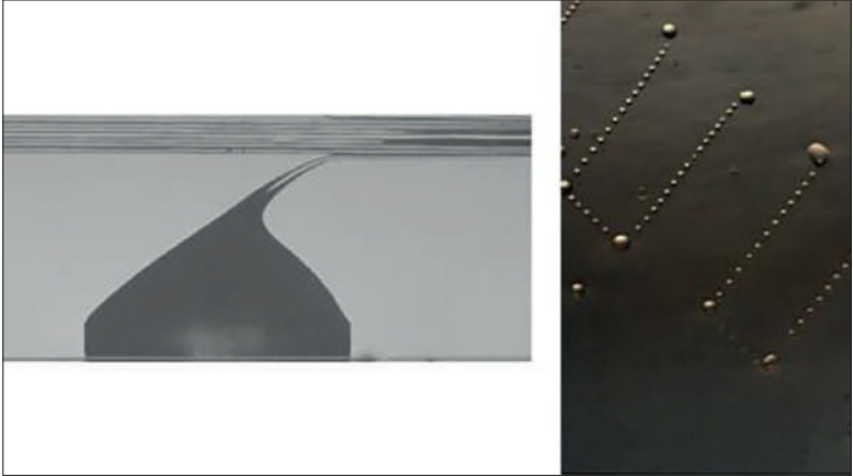
Stampa a getto piro-elettroidrodinamica senza ugelli di bioinchiostri senza buffer.
