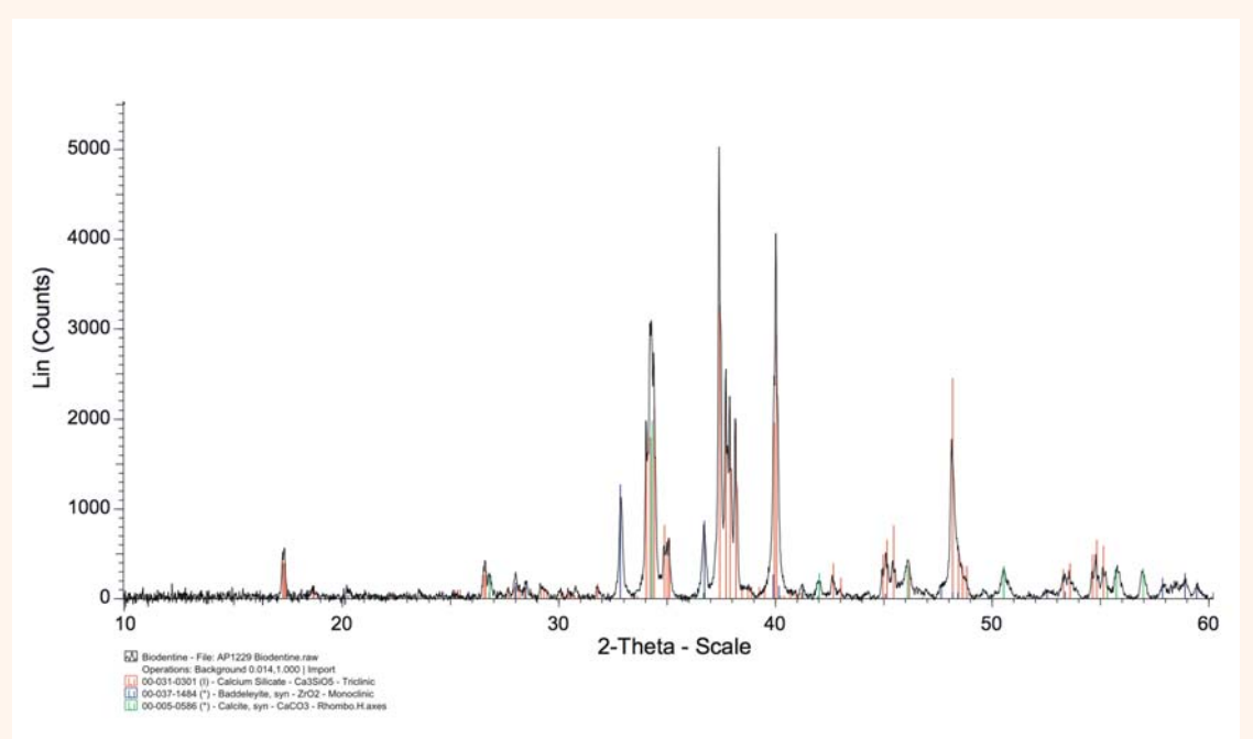
Fig. 2: Analiză cu difracția razelor X a pulberii Biodentine pentru a arăta principalele faze constitutive și anume silicatul tricalcic, oxidul de zirconiu și carbonatul de calciu. (Reprodus cu permisiune din Camilleri et al. 2013.)
