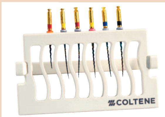
Рис. 5. Файлы HyFlex CM в последовательности их использования.
