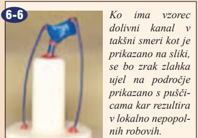
6-6 Ko ima vzorec dolivni kanal v takšni smeri kot je prikazano na sliki, se bo zrak zlahka ujel na področje prikazano s puščicama kar rezultira v lokalno nepopolnih robovih.
