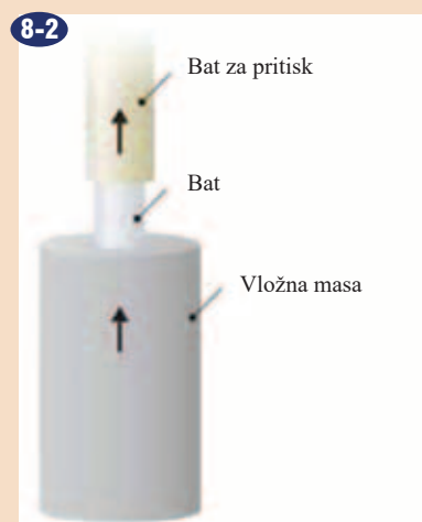
Ko je prešanje končano, bat za pritisk dvigne bat in povzroči srkanje že prešane keramike.
