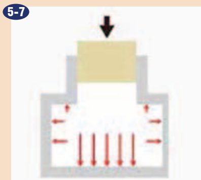
Shema pritiska prešanja. Pritisk se bolj izvaja v vertikalni smeri. Zaradi tega morajo imeti prešani izdelki dolivne kanale, da so robovi v njihovi smeri.
