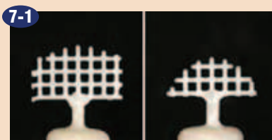
Levo - z odvodi; desno - brez odvodov. Odvodi, ki jih postavimo na zadnje točke, ki jih doseže prešana keramika, kot je prikazano na sliki 5-6, pomagajo odstraniti rezidualni zrak in naredijo razliko pri rezultatih prešanja, kot je prikazano zgoraj, tudi pri enakih pogojih.
