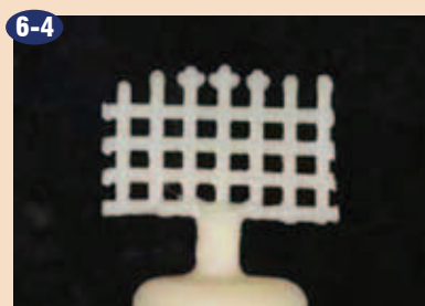
Idealno prešani pogoji v mrežastem vzorcu (vzorec iz voska iz GEO retencijske mrežice, vložna masa Renfert in dolivni kanal R25 so bili uporabljeni).
