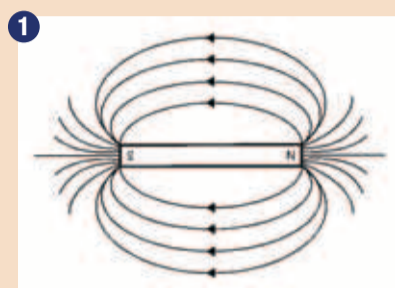
Magnetno polje
