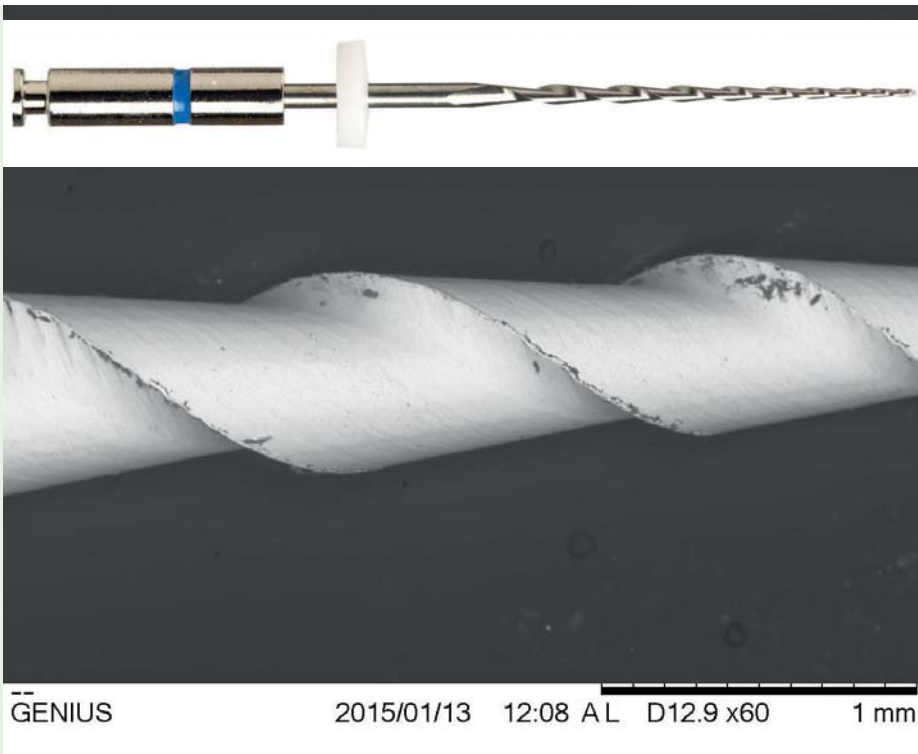
Fig. 5 : Grossissement d'une lime Genius, spiralée à l'endroit (© Dr Carlos Spironelli Ramos).
