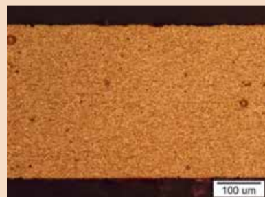
Vzdolžni prerez
