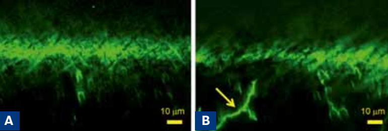
Figuren 3a & b: OP-controlegebied 6 µm onder het oppervlak (a). OP-behandeld gebied 10 µm onder het oppervlak (b). De pijl laat de scheur zien.
