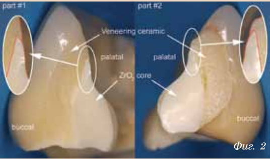
Фиг. 2: Счупване на керамичен ZrO 2 мост. Скелетът е намален от палатинално (прекомерно изразена капковидна форма), като не поддържа адекватно керамичните наслойвания. Прекалено големи размери на керамичните слоеве са станали обект на сили на опън. (Снимковият материал е любезно предоставен от проф. Улрих Лохбауер, Германия.)
