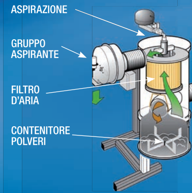
L'interno di un abbattitore di polveri per: sabbatrice, box ritocchi, rapide e pulitrici
