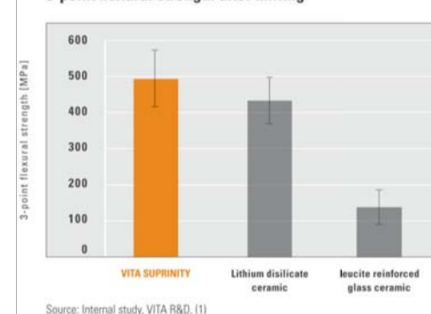
* Рис. 2: После шлифования у образцов из VITA SUPRINITY наблюдается более высокая прочность при 3-х точечном изгибе, чем у образцов из других керамических материалов. Источник: внутреннее исследование, VITA F&E
