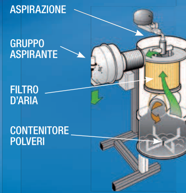
L'interno di un abbattitore di polveri per: sabbatrice, box ritocchi, rapide e pulitrici
